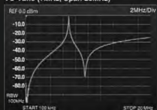
VC-Tune (7MHz, Span 20MHz)
