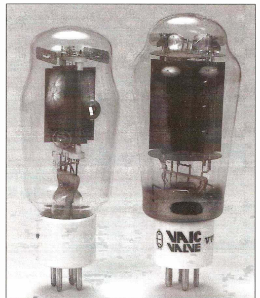
Svetlana SV811 and VAIC VV30B
