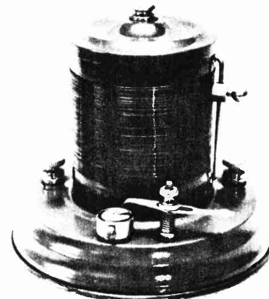
FIG.1 PANDORA CRYSTAL SET
