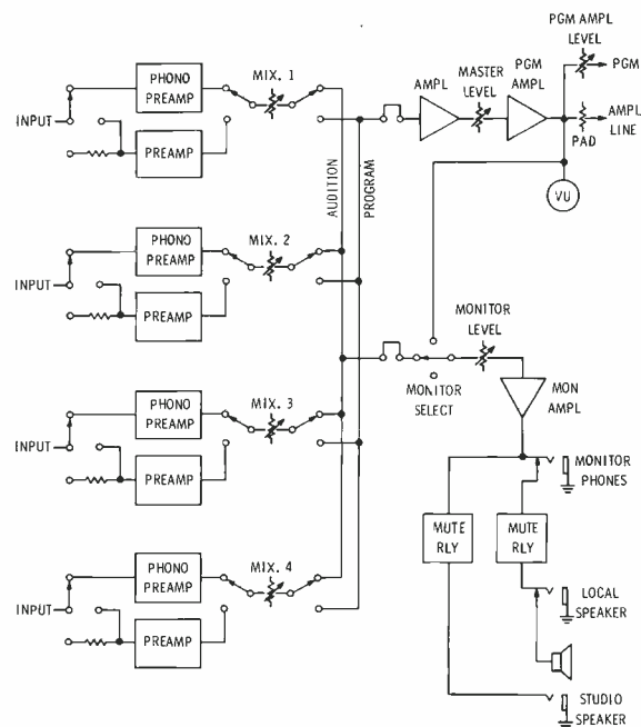
BLOCK DIAGRAM 212J-1
