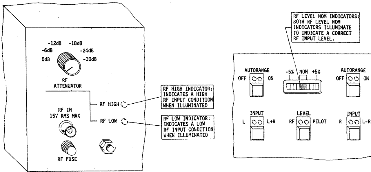
RF LEVEL NOM INDICATORS
