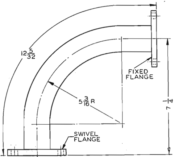
90° COUPLING MI-19310-2
