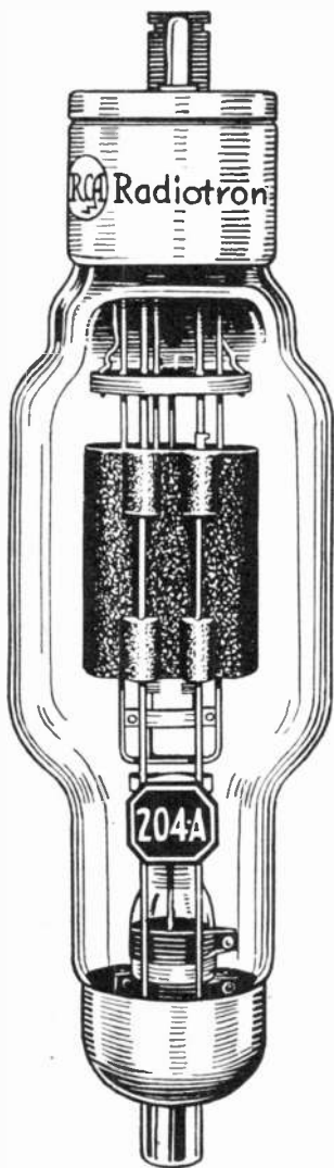
RCA-204-A
