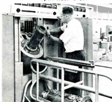
Tilt Klystron
