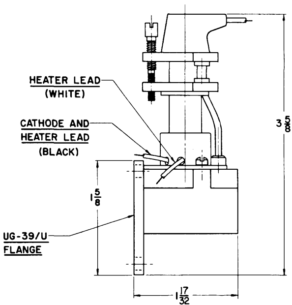
1K015XG (WAVEGUIDE OUTPUT)
