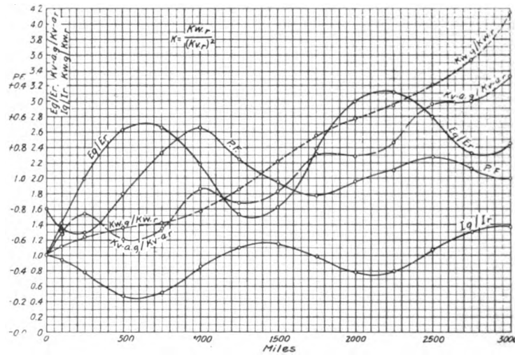
Fig. 27. 60 Cycles. K=5 , 0.8 Power-factor Lagging
