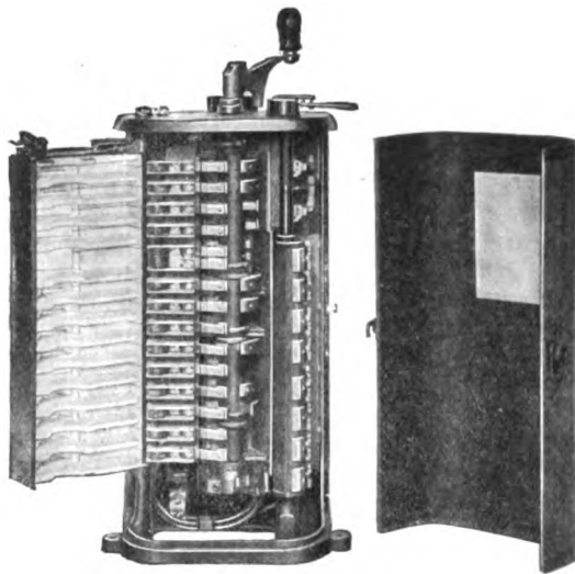
Fig. 9. K35 Controller
