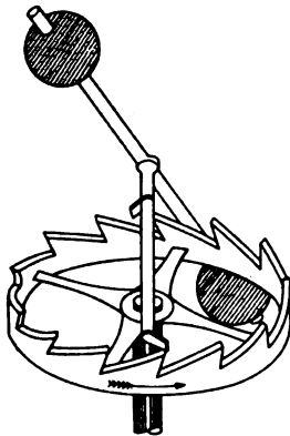
Fig. 3. Verge Escapement
