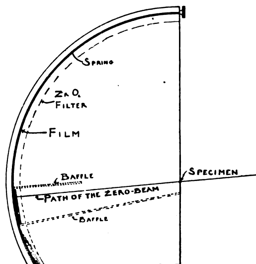
Fig. 6. Cassette
