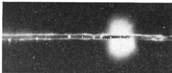
Fig. 20. Corona at 800-kv. 1-in. (2.54 cm.) Diameter Tube 144-in. (366 cm.) Spacing
