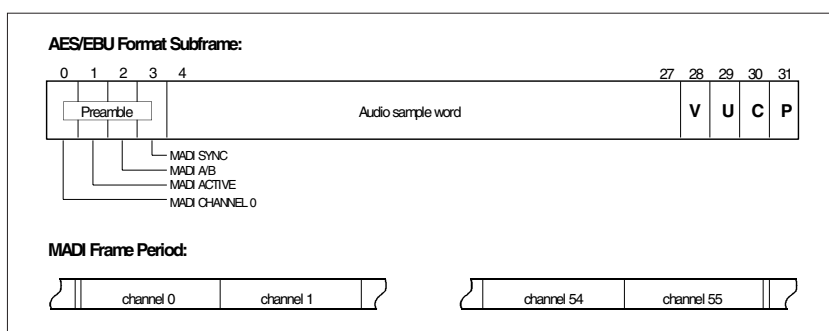
Fig. 2: MADI-Format
