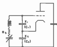
Fig. 2—Fundamental circuit.
