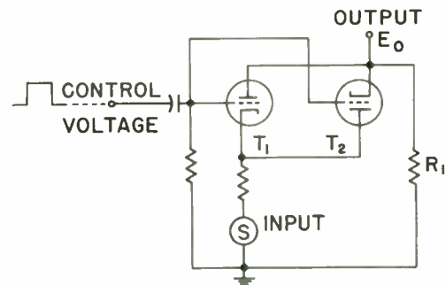
Fig. 1—A linear gate using triodes.
