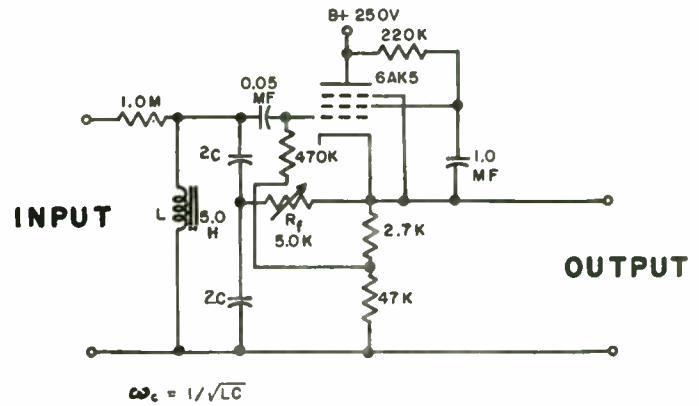
Fig. 5— Q multiplier.
