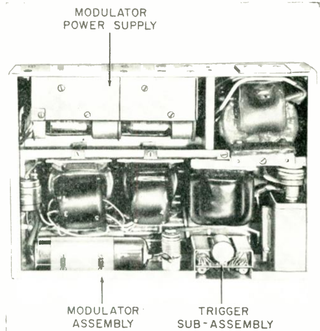
Fig. 7—Modulator.
