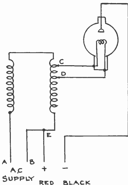
Fig. 8. Rectifier Connections
