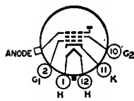
12D ANODE = O_3 + CL
