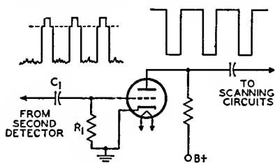
Fig. 42—Sync-separator circuit.
