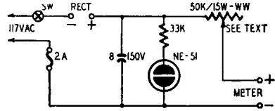
Fig. 127. Selenium rectifier tester.
