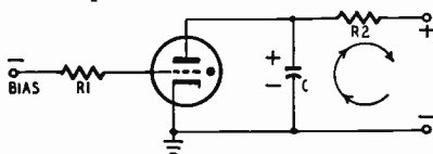
Fig. 304. Gas-tube sawtooth generator.
