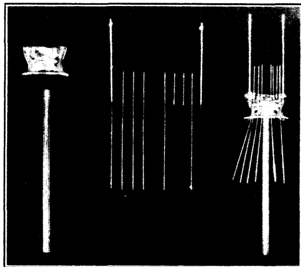
Fig. 1 - Glass-flare stem.
