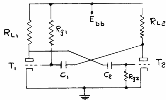
FIG. 17. Grid return circuit.
