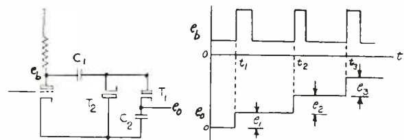
FIG. 28. Step-charging circuit.
