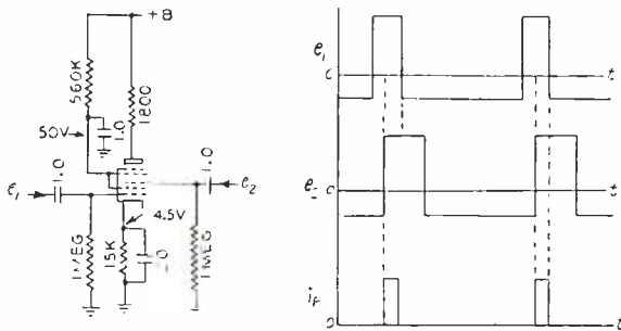
FIG. 29. Non-linear mixer.
