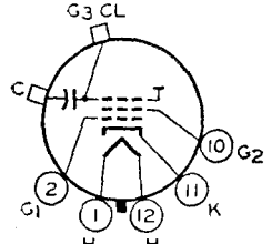
12N ULTOR = G_3 + CL
