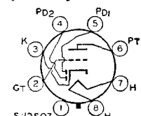
S:12SQ7 BC:12SQ7-GT
