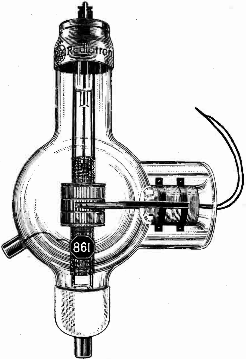
RCA-861
