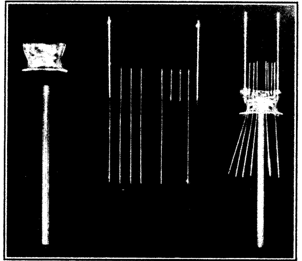
Fig. 1 - Glass-flare stem.
