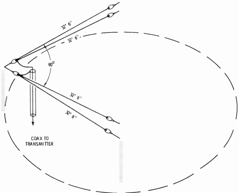
Fig. 56. 15-40 conical vee.
