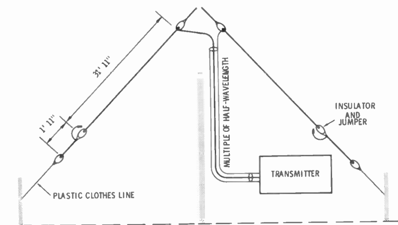
Fig. 35. Novice 15-40 inverted-vee antenna.
