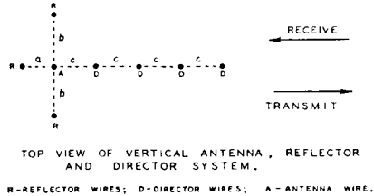
Fig. 48 Yagi Antenna.
