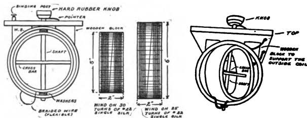
Fig. 161. Variometer.
