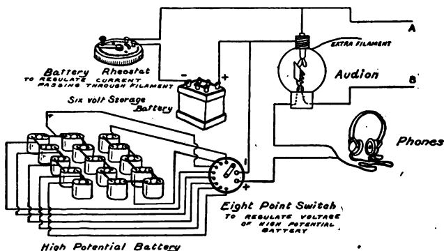
Fig. 166. Audion Circuit.
