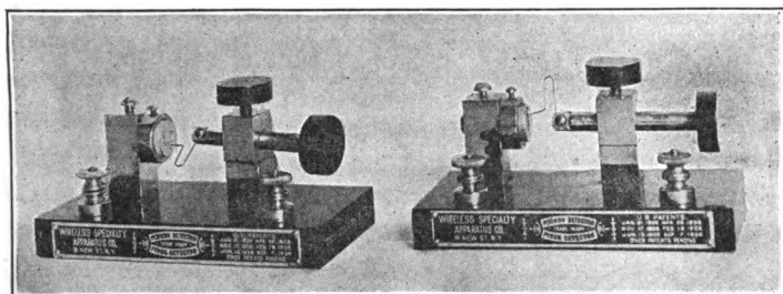
Fig. 163. Pyron Detector.
