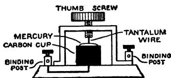
Fig. 103. Tantalum Detector.
