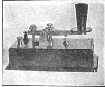
FIG. 219.—MARCONI KEY.
