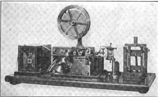
FIG. 212.—BEANLY-POPP RECEPTOR.
