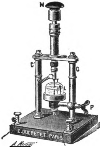
FIG. 222.—DUCRETET KEY.
