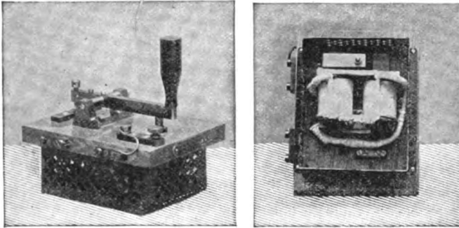
FIG. 220 a,b .—BRAUN KEY.
