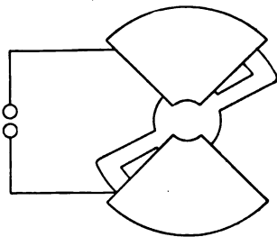
FIG. 139.—BJERKNÆS QUADRANT DETECTOR.
