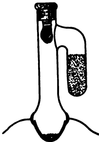
FIG. 147.— DUCRETET COHERER.
