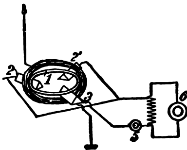
FIG. 151.— HERTZIAN DETECTOR. (Second Form.)
