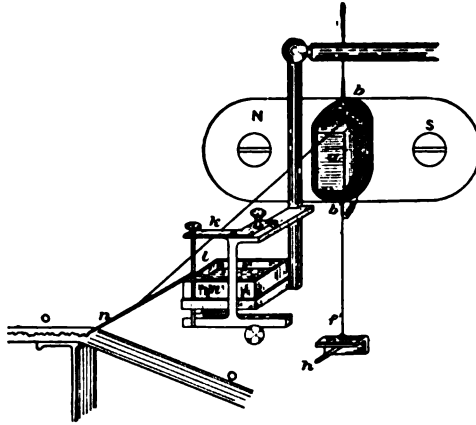
FIG. 246.—SIPHON RECORDER.
