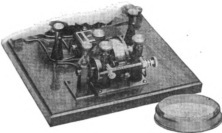
FIG. 236.—BRAUN DE-COHERER.
