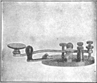
FIG. 218.—MORSE KEY.
