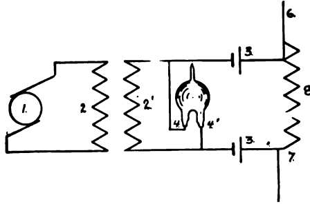
FIG. 123.—DIAGRAM MERCURY VAPOR INTERRUPTOR.
