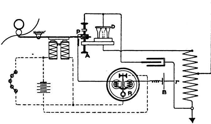
FIG. 211.—BRANLY-POPP RECEPTOR.
