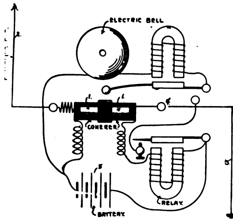
FIG. 190.—POPOFF RECEPTOR.
