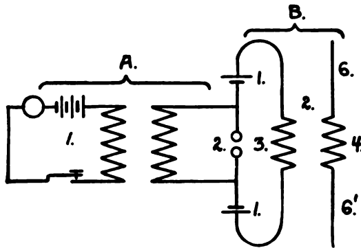
FIG. 176.—BRAUN TRANSMITTER.
