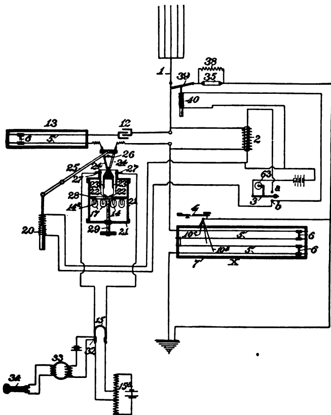
FIG. 204.—FESSENDEN SYSTEM.
