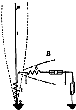
FIG. 195.—SLABY-ARCO RECEPTOR.
