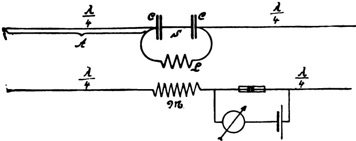
FIG. 197.—BRAUN RESONATOR.
