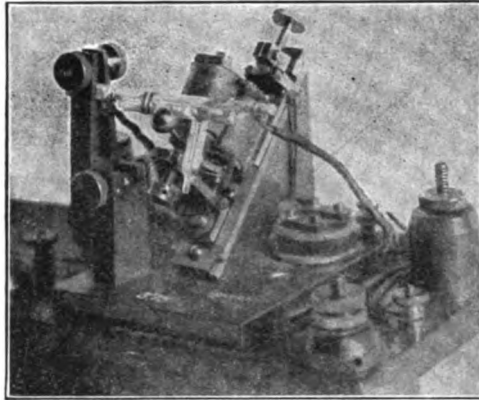
FIG. 235.—MARCONI DE-COHERER.
