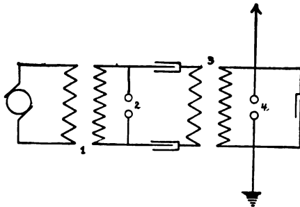
FIG. 127C.—TESLA OSCILLATOR.
