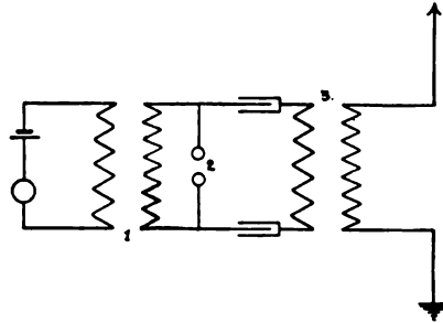
FIG. 127B.—BRAUN OSCILLATOR.
