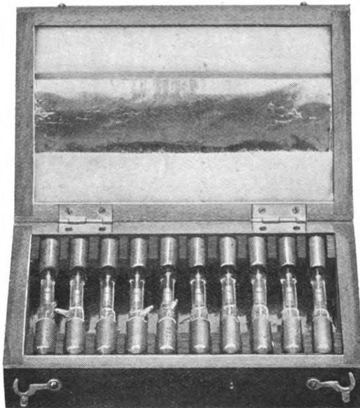
FIG. 52.—Coherer.
