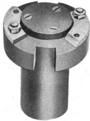
FIG. 53.—Schloemilch Detector.
