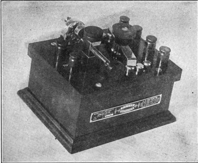
FIG. 70.—Perikon detector.
