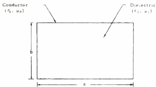
Figure 2-15. Waveguide Parameters
