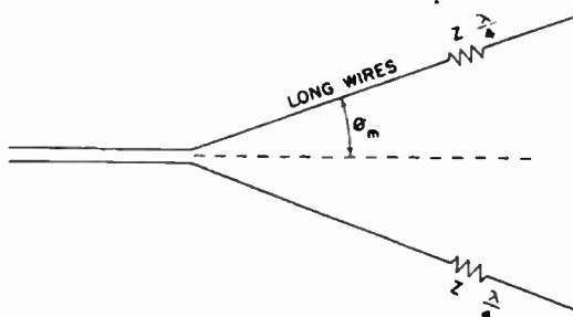
FIG. 3.74. Traveling-wave V antenna.
