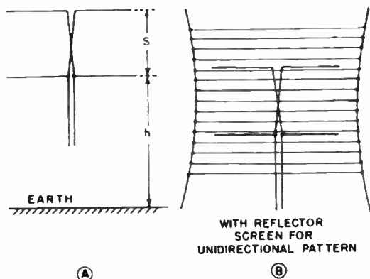
FIG. 3.48. Lazy-H antennas.
