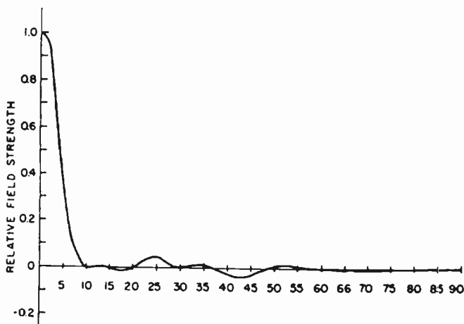
FIG. 3.59. Array horizontal pattern.
