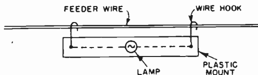
FIG. 4.61. Miniature-lamp indicator.
