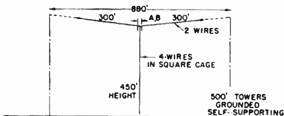
FIG. 1.30. Inverted-L antennas.
