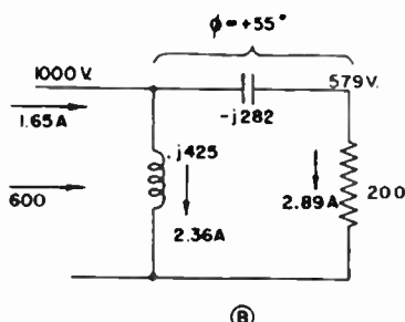
Fig. 2.27. Network B .
