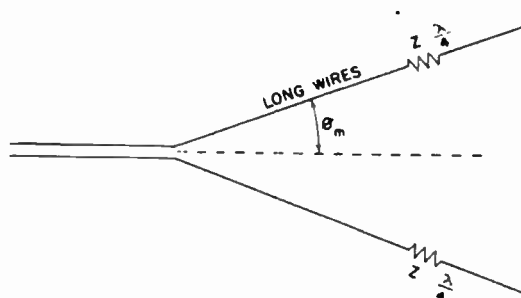
FIG. 3.74. Traveling-wave V antenna.
