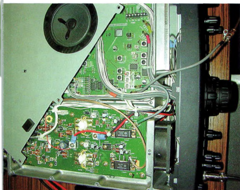
Une vue « aérienne » de l'intérieur du FT-847 et le câble gris là droite qui part vers l'entrée du modulateur. La partie supérieure de l'image montre qu'il est possible d'intégrer le module définitif dans le transceiver.
