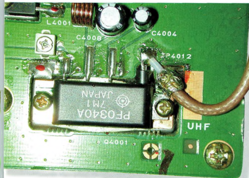
On voit ici en gros plan l'étage d'entrée de l'amplificateur de puissance. Le câble Téléphon qui y arrive part vers la sortie de notre modulateur d'amplitude universel.
