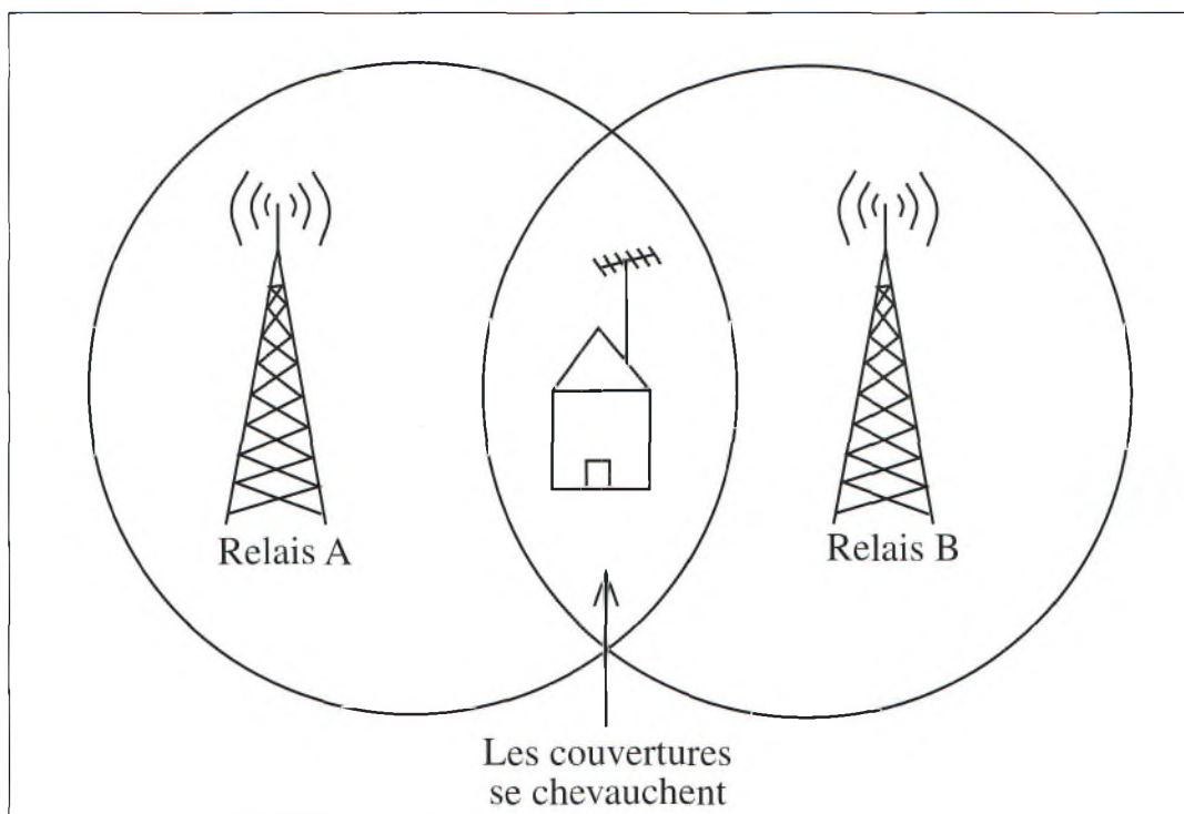
Fig. 1- La couverture des deux relais se chevauche. Cela peut être dû à la propagation par exemple. L'emploi du CTCSS permet d'éviter les déclenchements mutuels des deux relais.
