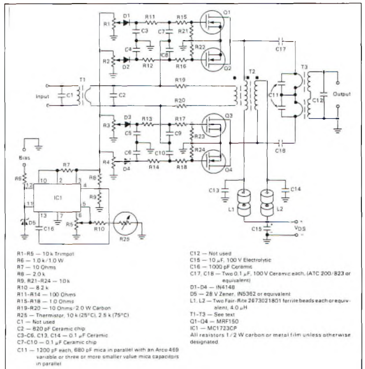
Le schéma d'application proposé par Motorola.
