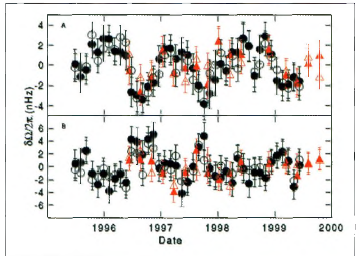
Fig. 2- Variations temporelles de la différence de la vitesse de rotation des couches à 0,72 R et à 0,63 R plus bas. Les résultats ont été observés par deux équipes, différenciées ici par les indications en rouge pour l'une, en noir pour l'autre.
