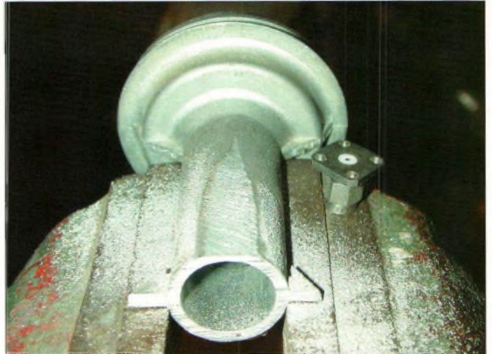
Fig. 3-On doit pratiquer un méplat sur la circonférence du guide pour faire tenir l'embase du connecteur SMA.
