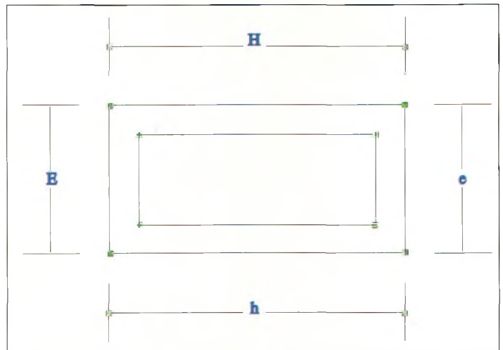
Vue frontale et dimensions d'un guide WR.
