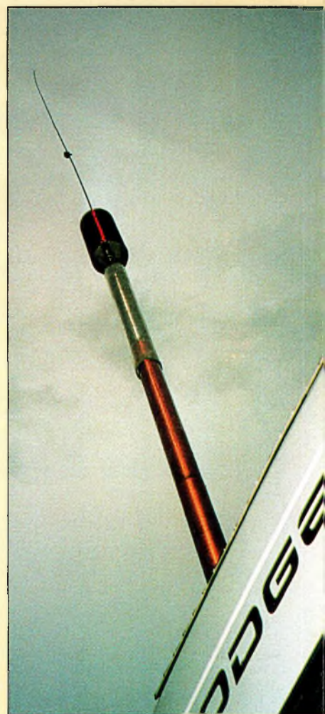
L'antenne (réduite II de KH6DX/M. Qui a dit qu'il fallait des grandes antennes pour cette bande ?
