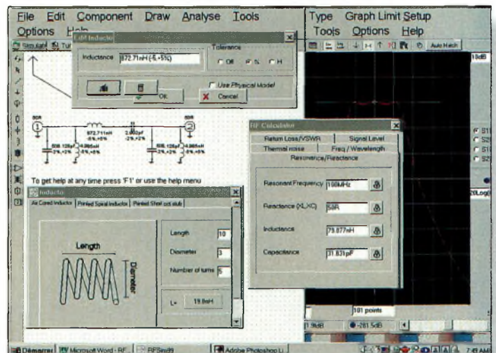
L'étude d'un filtre sur 145MHz à partir de celui d'origine.
