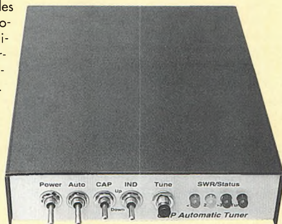
Photo D- Ce tuner d'antennes automatiques LDG autonome est l'un des nombreux appareils fabriqués pour fonctionner avec tous les types de transceivers et il rend les opérations "mains libres" très faciles. Cet appareil comprend aussi un pont SWR intégré pour la commodité.
