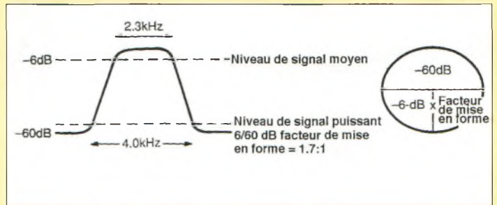
Fig. 1 - Les fabricants utilisent souvent les courbes de réponse FI comme celles-ci pour décrire la sélectivité FI de leur transceiver avec des filtres SSB ou CW quartz ou céramiques intégrés ou optionnels. (Voir texte)
