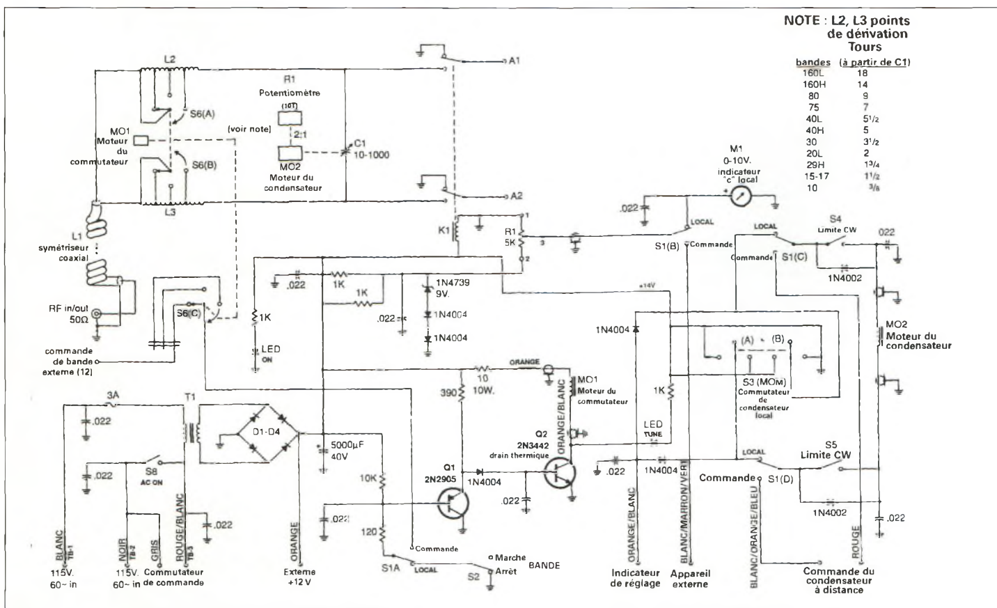
Fig. 3 - Schéma du circuit du tuner.
