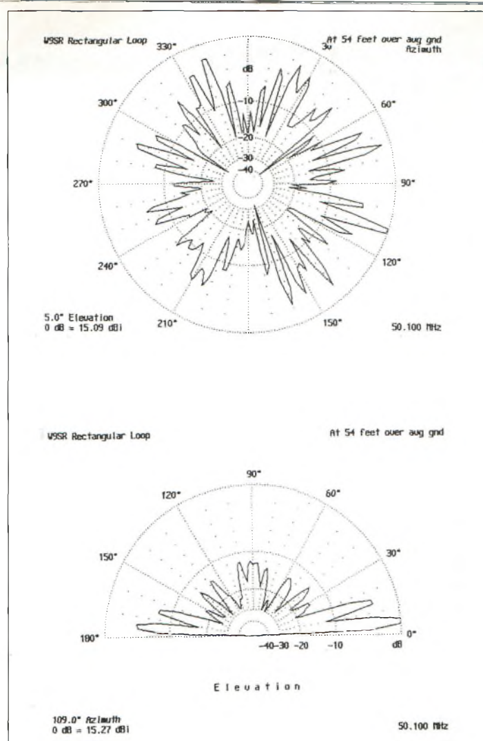
Fig. 1(H)- Rayonnement en horizontal et vertical sur la bande des 6 mètres.
