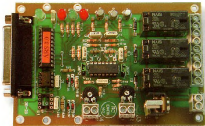
Les borniers reçoivent la connexion des fils du rotor. Notez les quatre LED qui affichent le sens dans lequel tournent les antennes.
