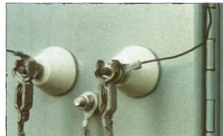
La mise à la terre est assurée par des pinces accrochées directement en sorties des isolateurs.
