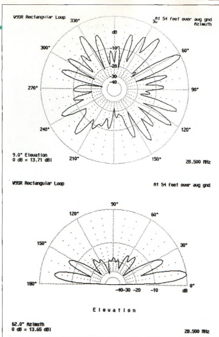
Fig. 1(G)- Rayonnement en horizontal et vertical sur la bande des 10 mètres.
