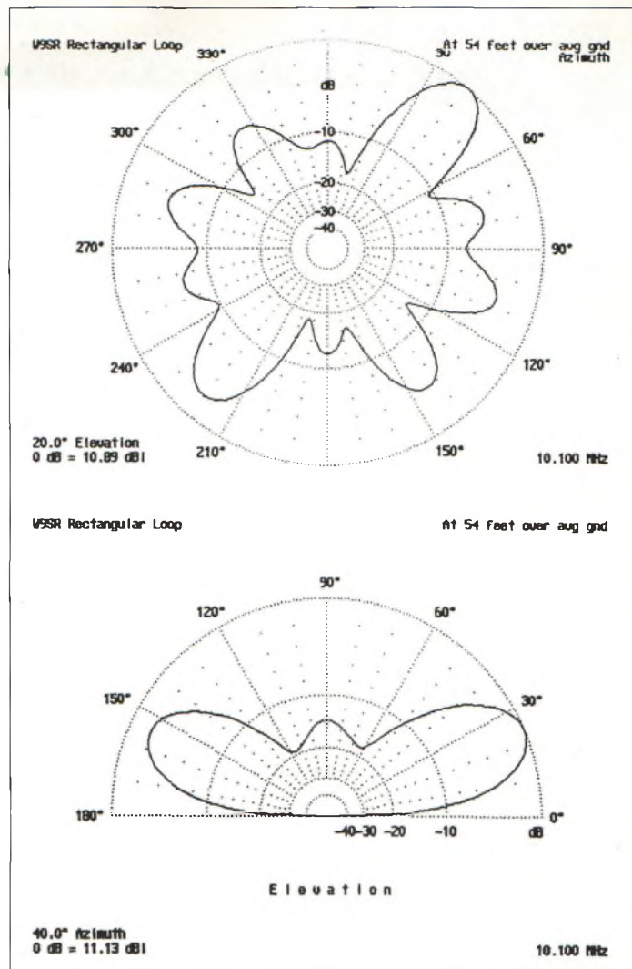
Fig. 1(D) - Rayonnement en horizontal et vertical sur la bande des 30 mètres.
