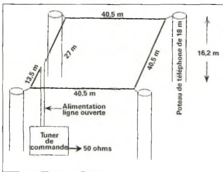
Fig. 2 - Dimensions et disposition de l'antenne cadre réglée.
