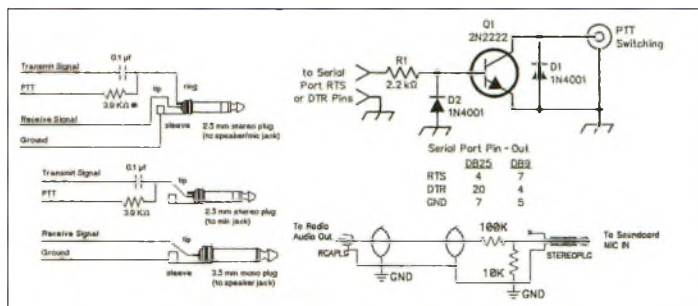
Les schémas pour mettre en œuvre électroniquement un système APRS à partir de la carte son. Il est à noter que ces mêmes montages fonctionnent pour la SSTV.
