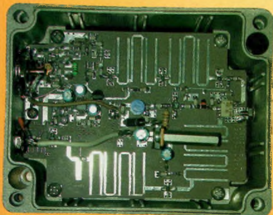
Pleins feux sur le convertisseur de Downeastmicrowave : Une réalisation sans souci d'après Mattieu, F4BUC.
