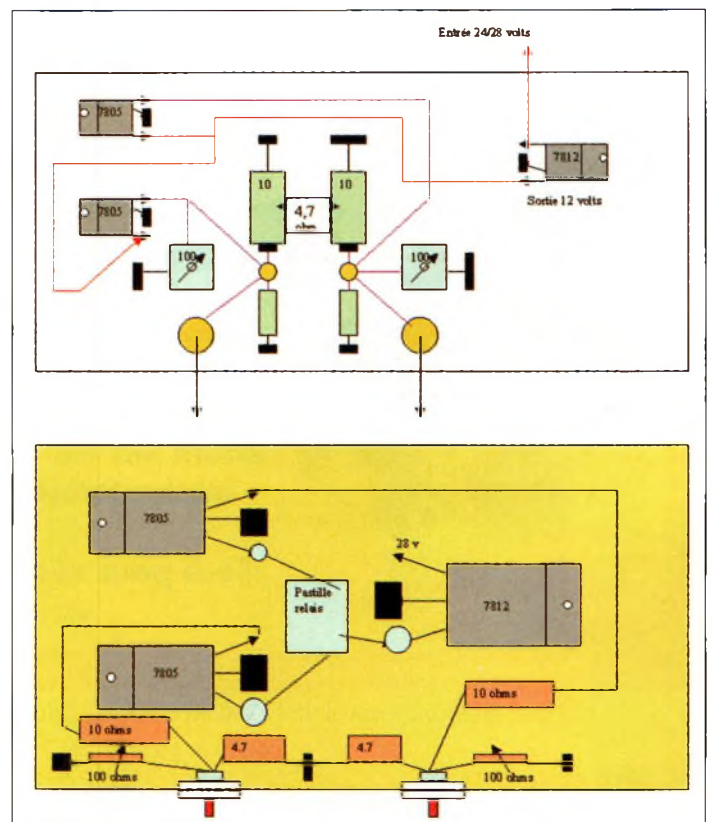
Fig. 1 - Disposition et implantation des éléments sur la plaquette.
