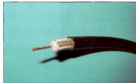
Le câble du RG-213 est délicatement dénudé avec un cutter.
