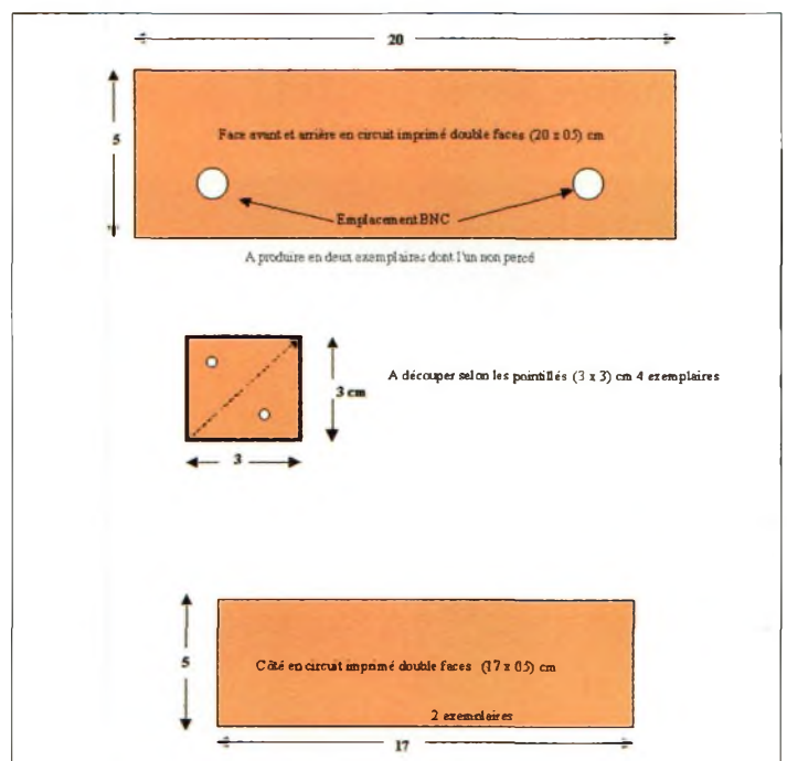
Fig.4- Plan de découpe des façades époxy.
