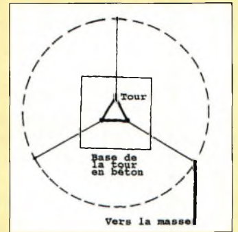
Fig. 1- Mettre à la terre correctement votre pylône est un point important.
