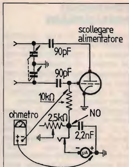
figura 2 Controllo ohmetrico della sezione oscillatrice del GDM. Evitare di collegare l'ohmetro fra il punto "NO" e massa, potrebbe passare una corrente distruttiva nel microamperometro. Il controllo ohmetrico comprende anche la verifica di isolamento dei vari capacitori e degli elettrodi della valvola che sono anch'essi... capacitori.
