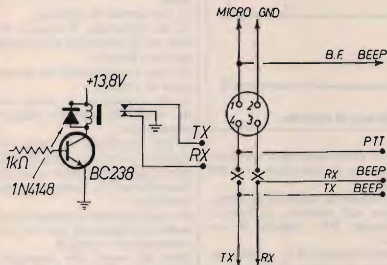
figura 5 Schema di commutazione alternativo e relative connessioni.
