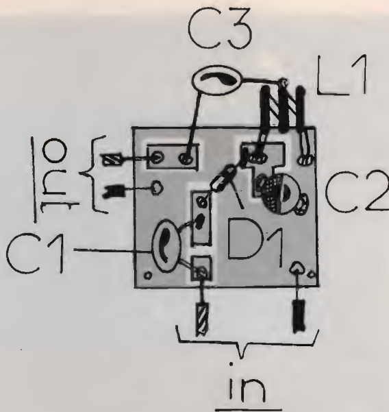
figura 3 Piano di montaggio del moltiplicatore di frequenza.
