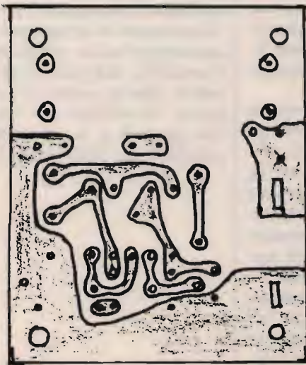
figura 2 Circuito stampato del ricevitore tascabile per Onde Medie.
