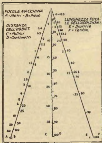
FIG. 3 - Questo semplice grafico vi consentirà di calcolare agevolmente la lunghezza focale, conoscendo la potenza in diottrie di una lente, e le diottrie, conoscendo la lunghezza focale Riproducetelo su di un cartoncino e conservatelo, perché vi sarà utilissimo in mille occasioni.
