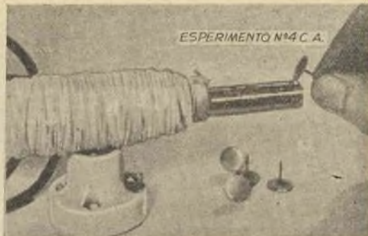
In una barra di acciaio magnetizzata per mezzo della corrente continua il magnetismo scompare per effetti delle continue inversioni di senso del campo prodotto da una corrente alternata.
