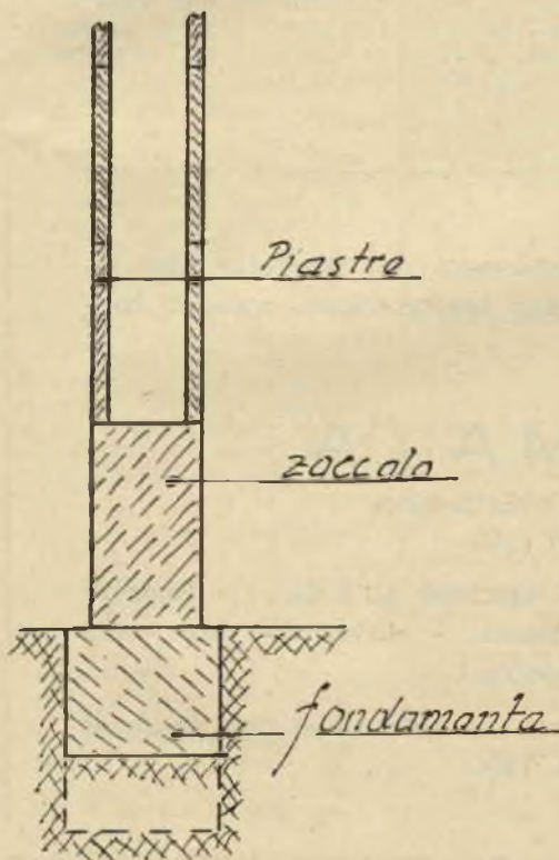
sez. B-B.
