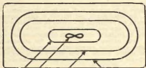
CATODO FILAMENTO GRIGLIA CONTR. GRIGLIA SCHER. PLACCA 37
