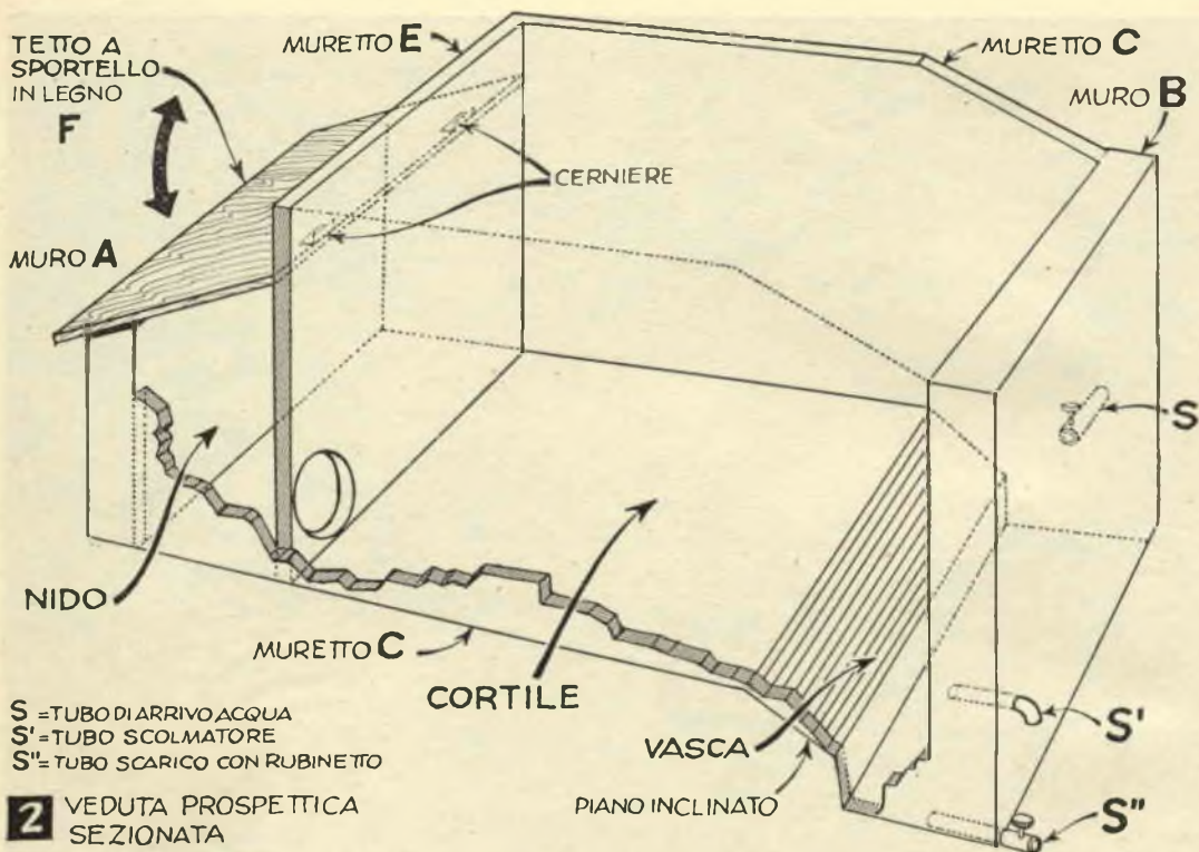
2 Veduta prospettica sezionata di nido per una famiglia di nutria. Notate il tubo «S», che impedisce all'acqua di raggiungere il piano del «cortile» ed il nido propriamente detto.
