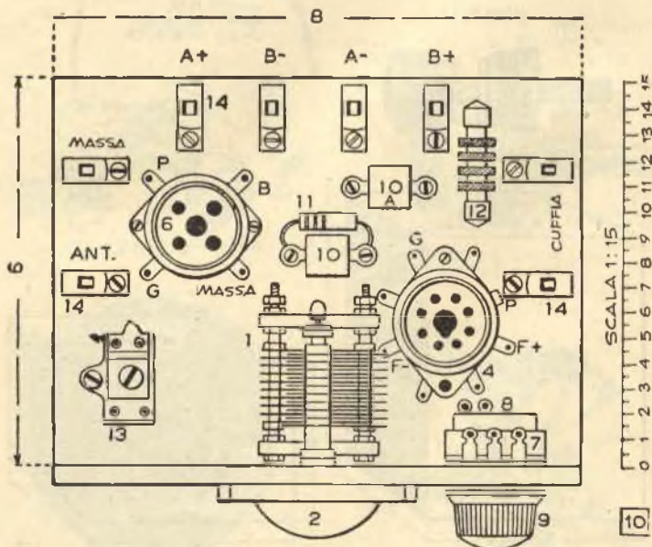
Fig. 10 - Come vanno disposti i componenti dell'apparecchio sulla base del telaio. Chi lo desidera può servirsi della nostra scala per determinarne l'esatta posizione.
