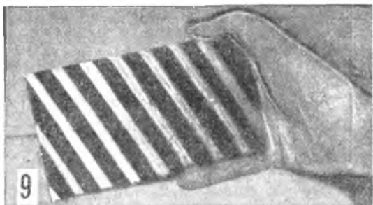
Un esempio di superficie di alluminio anodizzata e successivamente colorata. Per questo lavoro mi sono servito di nastro tipo Scotch Tape e di vernice di riserva.
