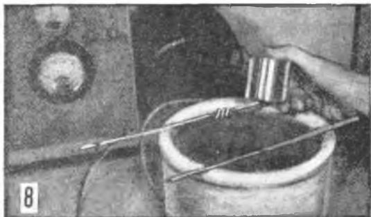
Recipiente per la detersione e per l'anodizzazione. Le barrette esterne che sostengono i catodi e gli anodi debbono essere di rame o di ottone.
