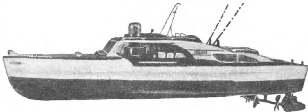
Veduta laterale, illustrante il complesso dello scafo e della sovrastruttura, uniti.
