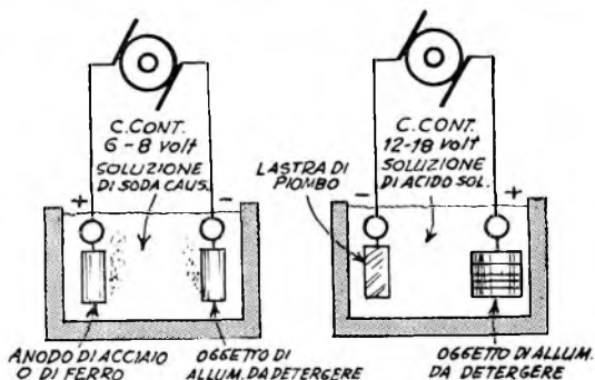
Recipiente per la detersione e per l'anodizzazione. Le barrette esterne che sostengono i catodi e gli anodi debbono essere di rame o di ottone.
