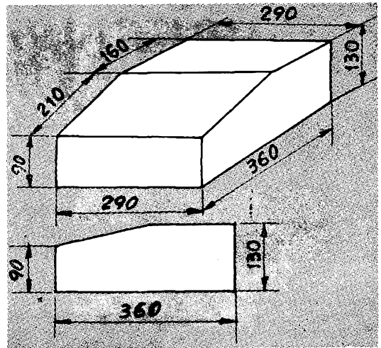
Dimensioni, forma e misure in centimetri della cassetta contenente il provavalvole.
