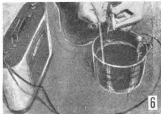
L'oggetto, afferrato da un clip o da un morsetto, a sua volta collegato al polo negativo della batteria (a 6 volt), fungerà da catodo, durante il processo della deposizione.
