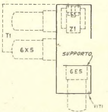
VISTA LATERALE CON SUPPORTO 6E5 MONTATO
