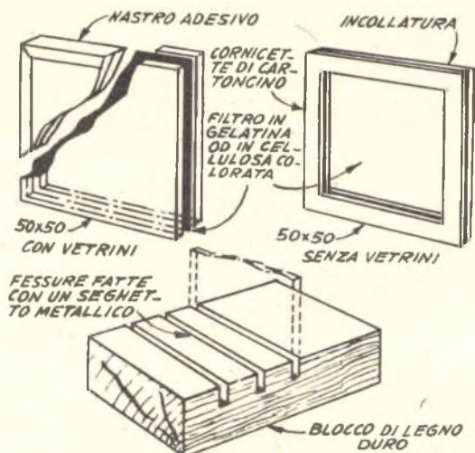
Illustrazione dei metodi per montare dei filtri colorati in cornicette di cartoncino o tra lastrine di vetro.
