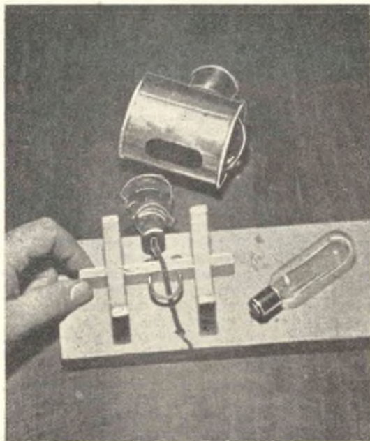
Sistema per lo scorrimento della lampada, per la messa a fuoco di questa ultima. Il listellino centrale di legno scorre liberamente attraverso le scanalature praticate nei due pezzi di legno formanti la culla per la lanterna. La vite ad "U" serve per trattenere il portalampane sul listello. Le lampade di questa foto sono state ambedue provate, con ottimi risultati.
