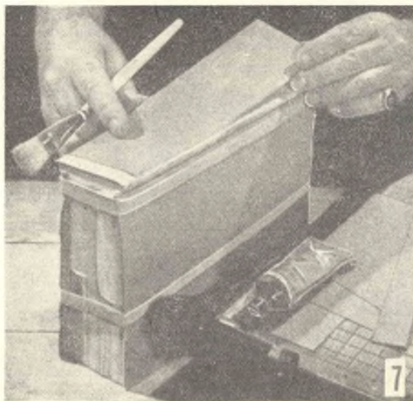
FIGURA 7 - Incollare una striscia di carta pesante, colorata, delle dimensioni della costola, al di sopra della garza. La lunghezza della carta dovrà essere tale che non abbia a coprire le due striscette di cimosa. FIGURA 8 - Montare un poco di cartavetro su di un blocchetto di legno mezzorotondo, e con questo lavorare sulla parte delle pagine opposte a quella della costola, per conferire all'insieme di esse una certa concavità. Per ottenere ciò, necessita, naturalmente, agire principalmente sulla parte centrale del gruppo delle pagine.
