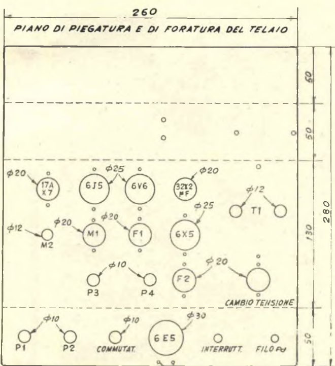
VISTA SUPERIORE PRIMA DELLA PIEGATURA
