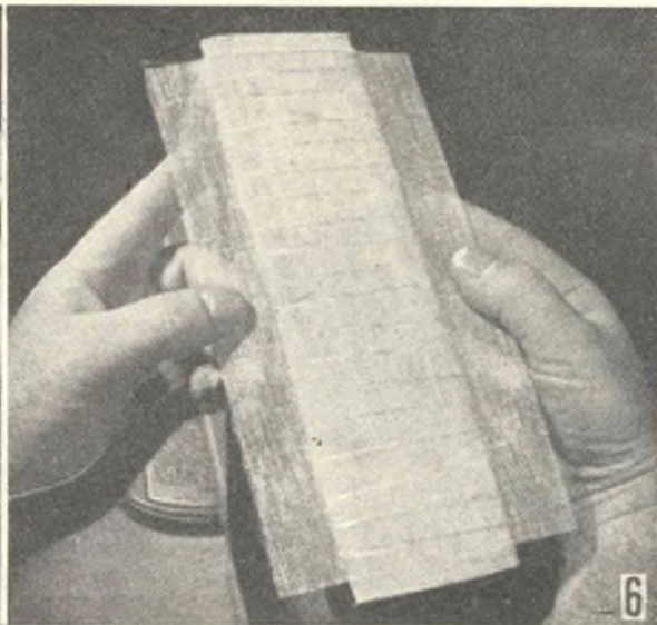
FIGURA 5 - Applicazione dei pezzetti di cimosa colorata, agli spigoli della costola. Essi vanno applicati soltanto dopo che l'intera costola del volume sarà stata coperta abbondantemente di mastice alla para, lasciata seccare e lisciata alla perfezione con cartavetro. FIGURA 6 - Prendere un rettangolo della garza apprettata di dimensioni tali che risulti in totale 25 mm. più corto e 50 mm. più largo della costola. Applicare un altro poco di mastice e premervi sopra la garza. Attendere l'essiccazione, poi togliere per un momento i cartoni, stendere sotto di essi la porzione sovrabbondante della garza e rimmetterli dopo avere applicato pochissimo altro mastice.
