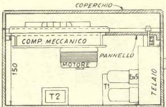
SEZ. LONGITUDINALE
