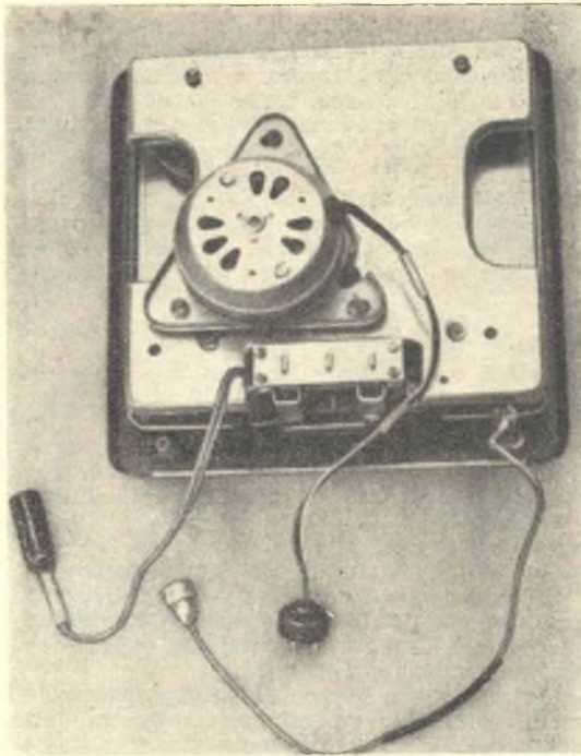
Il complesso meccanico visto di sotto.
