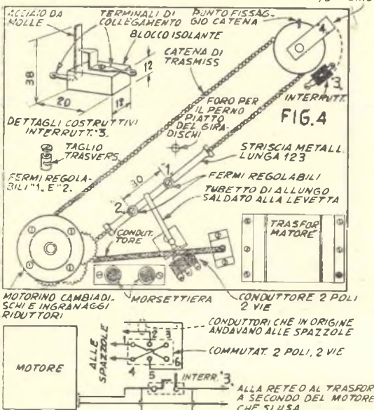
MECCANISMO DEL CAMBIADISCHI VISTO DAL DI SOTTO LA LEVA 4 APRE L'INTERRUTTORE DOPO AVER COMPIUTO 1/3 DI GIRO
