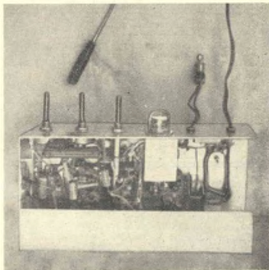
Il telaio « amplificatore-oscillatore-alimentatore » nella sua parte inferiore. Notare la sistemazione della 6E5.
