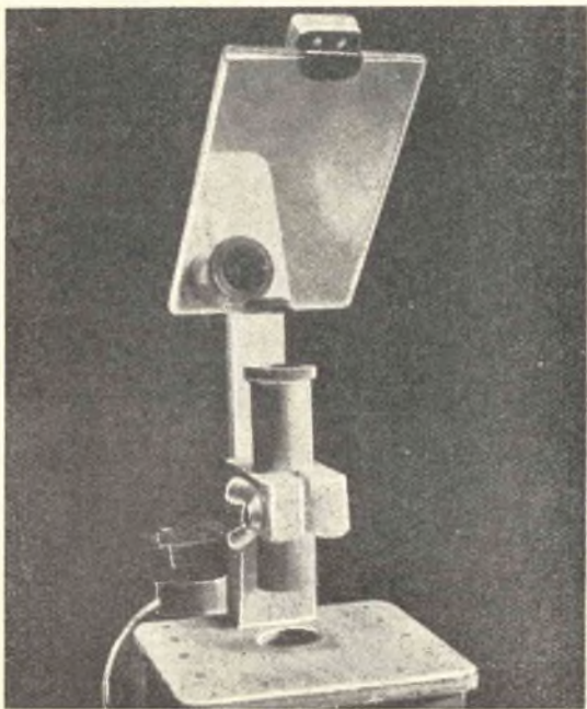
Piccole staffe di metallo trattengono lo specchio superiore sulla sua montatura. Funzione di questo specchio è quella di deviare in direzione orizzontale il raggio dell'immagine, altrimenti rivolto verso l'alto.
