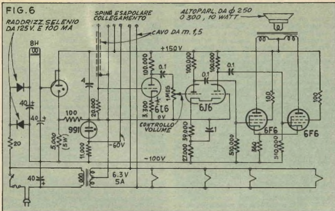
Completo comune dello strumento, composto dagli stadi di preamplificazione e di amplificazione finale nonché dai circuiti di alimentazione e di stabilizzazione della tensione. I sei fili che sporgono dalla parte alta del circuito elettrico vanno collegati nell'ordine ai sei conduttori del cavo esapolare che fa capo a ciascuna delle singole sezioni.
