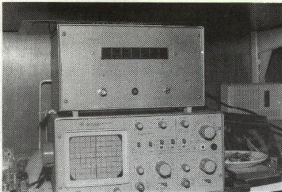
Studio VTA: Frequentieteller (boven) en oscilloscope (beneden).
