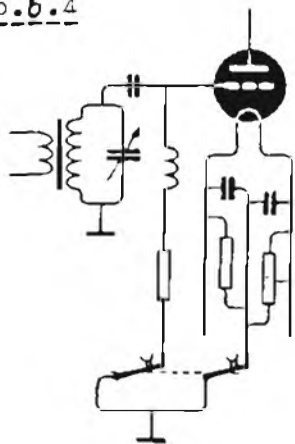
Sleutelen, tegeliker-tijd in roostercircuit en anodekring.
