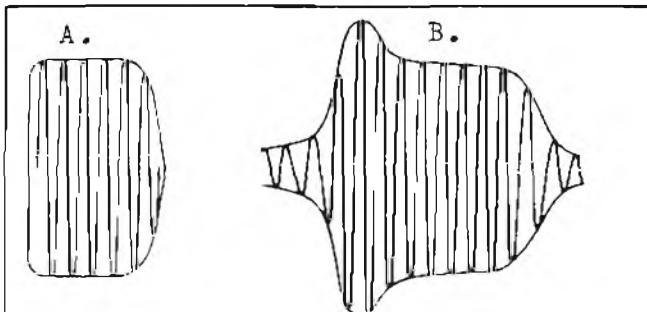
afb. 6.5. A, de ideale vorm van het seinteken. B. Ampl. zwelt aan en neemt af bij afloop seinteken.
