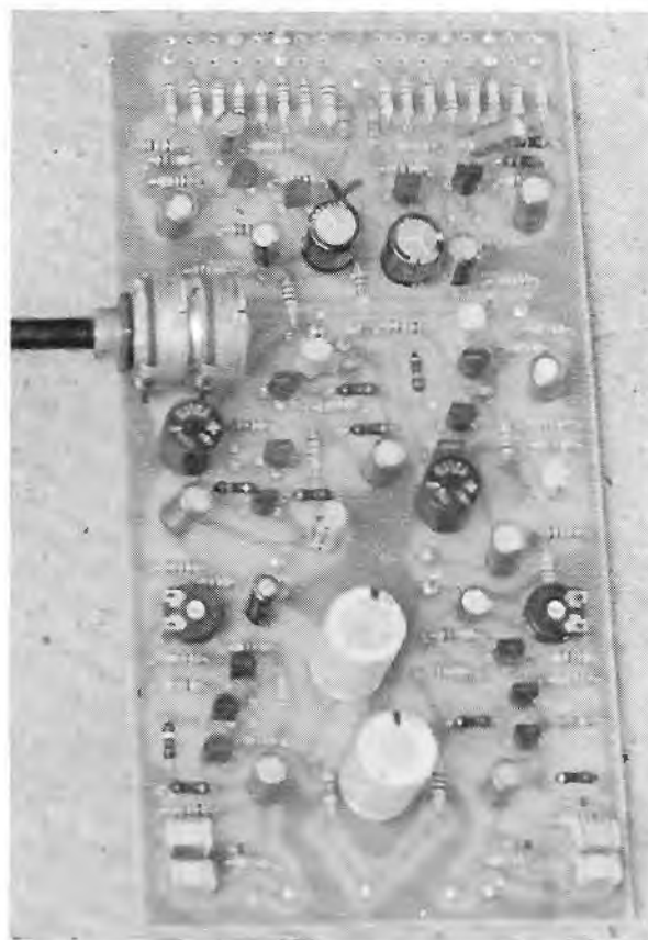
Lijnversterker/VU-metermoduul
