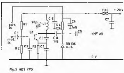
Fig.3 HET VFO
