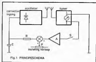
Fig. 1 PRINCIPESHEMA
