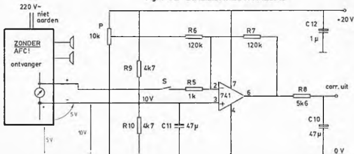
Fig.4 DE STABILISATIESCHAKELING
