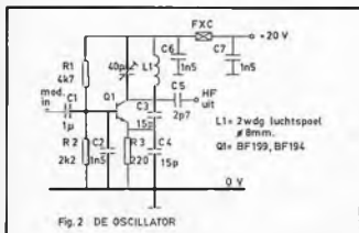
Fig. 2 DE OSCILLATOR
