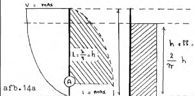
afb. 14 De Marcony-antenne, de verticaal opgestelde 1/4-straler. Daarnaast afgebeeld het elektrische vervangingsschema.
