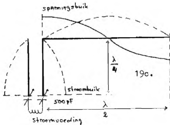
Afh.19: De Zeppelin-antenne, waarin een hele golflengte wordt gehalveerd in een 1/2 golf straler met een twee-draads voedingslijn die 1/4 golf (of veelvoud daarvan) lang moet zijn. Alleen dan treedt er stroomvoeding op. Voor harmonischen is spanningsvoeding in het koppelpunt nodig.
