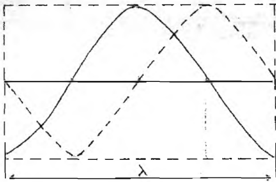
Afh.19: De Zeppelin-antenne, waarin een hele golflengte wordt gehalveerd in een 1/2 golf straler met een twee-draads voedingslijn die 1/4 golf (of veelvoud daarvan) lang moet zijn. Alleen dan treedt er stroomvoeding op. Voor harmonischen is spanningsvoeding in het koppelpunt nodig.
