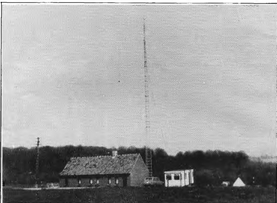
DE STUDIO'S EN ZENDMAST VAN RADIO INTERCITY (RESERVE-ZENDMAST LINKS VAN HET HUISJE)
